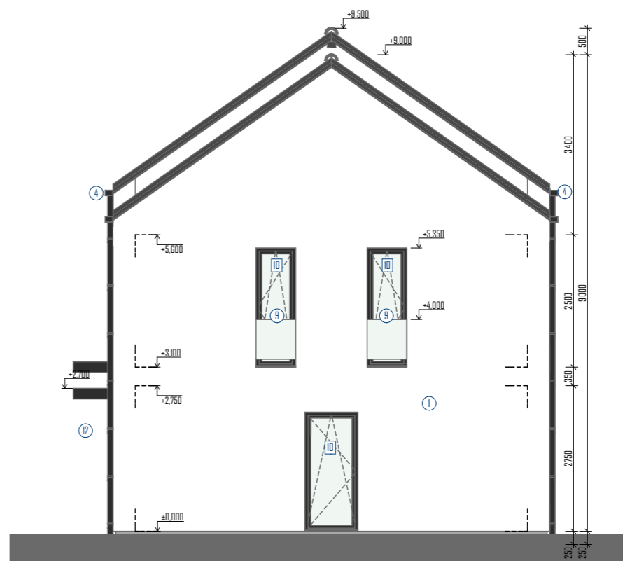
SO-102_POHLED SEVERNÍ
