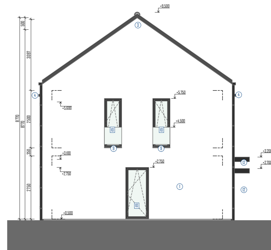
SO-102_POHLED JIŽNÍ
